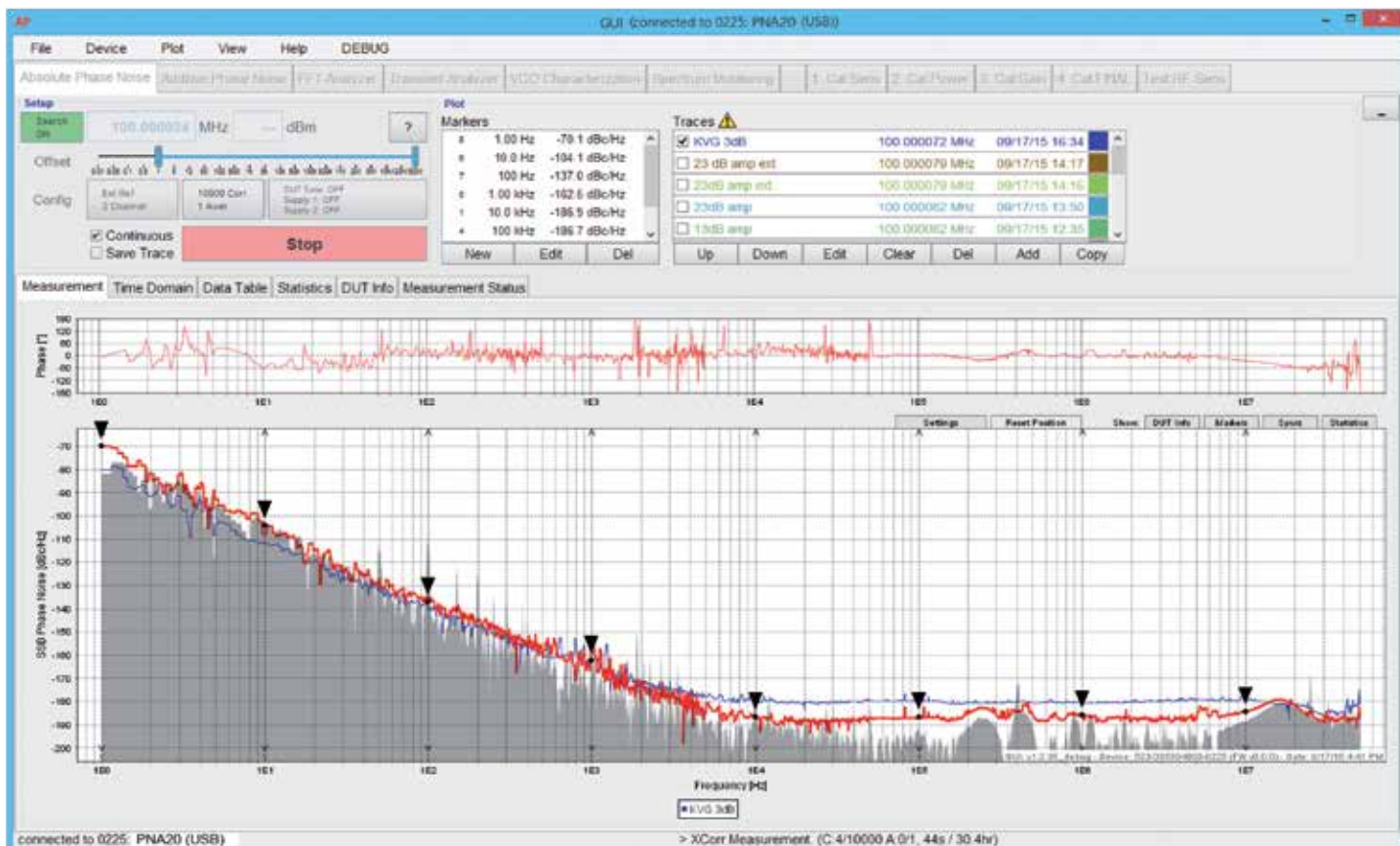
6 Интерфейс пользователя
